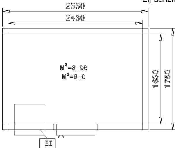
Zij aanzicht
